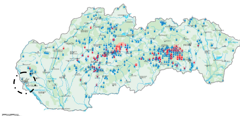
Obrázok: Kontaminácia pôd v okolí M.Č. Bratislava - Vajnory Zdroj: http://apl.geology.sk/atlaskrajiny/ , 2023
