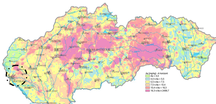
Obrázok: Výskyt Arzénu v pôde - A horizont v okolí M.Č. Bratislava - Vajnory
