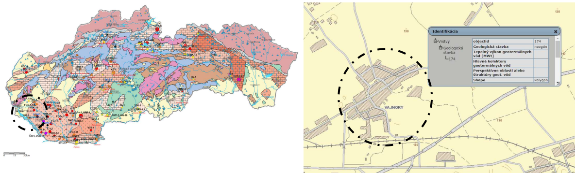
Obrázok: Zdroje geotermálnych a minerálnych vôd v mestskej časti Bratislava - Vajnory.
