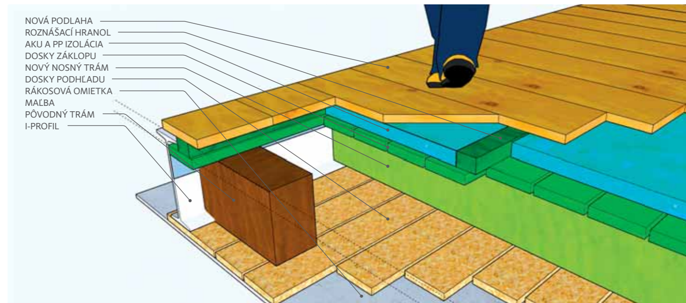
Obrázok č. 4 – Návrh nového zloženia stropu
